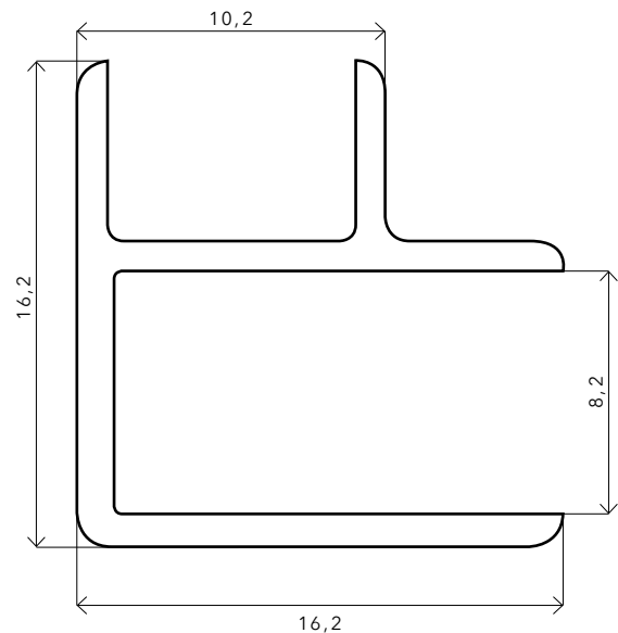
Profilquerschnitt Länge 3050 mm
