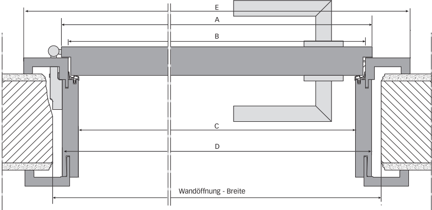
Holztürelement 2flg. gefälzt
