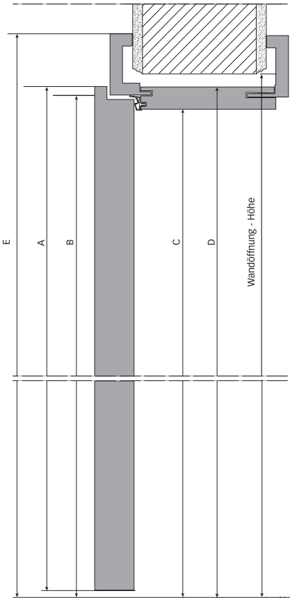
Holztürelement gefälzt
