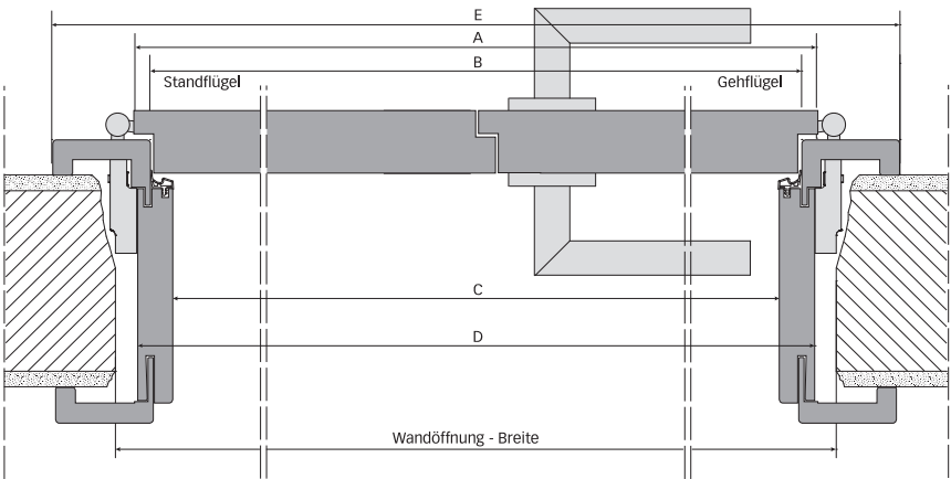
Holztürelement 2flg. gefälzt
